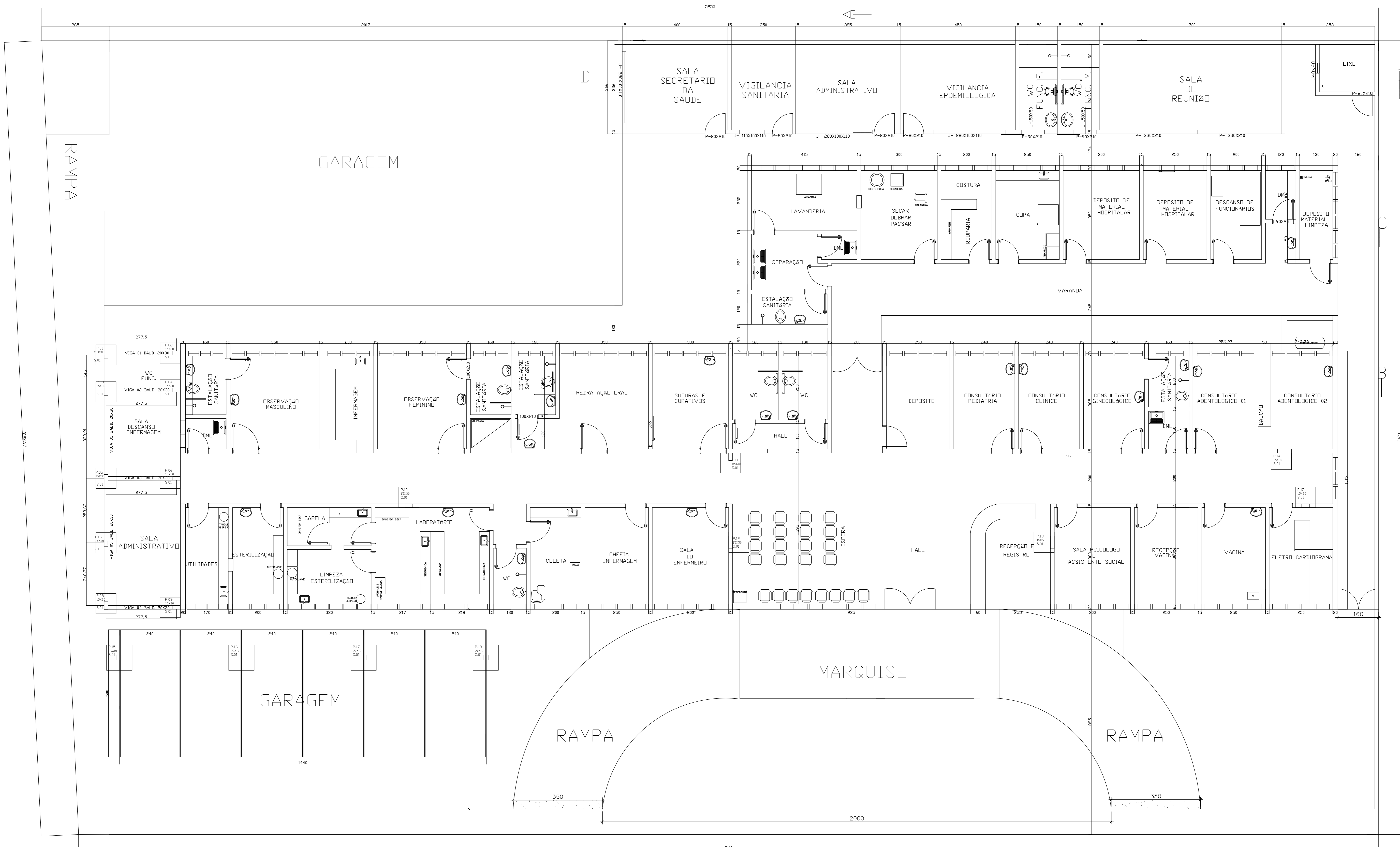
PLANTA BAIXA ESTRUTURAL ESCALA: 1/50
